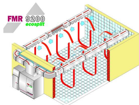
Abb. Räucherkammer
